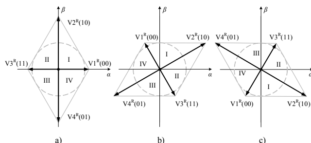
Rys. 2. Wektory możliwych do uzyskania napięć fazowych przekształtnika po załączeniu jednego z triaków: TrA (a), TrB (b) oraz TrC (c)
